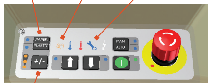
Einstellbare Ballengröße
